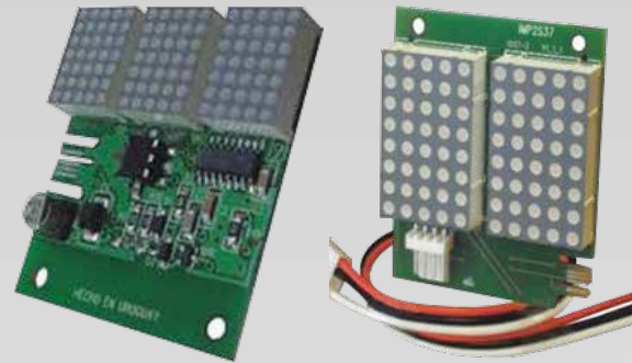
Displays de 37mm Matriz de Punto
